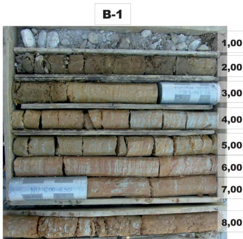
Slika 9. Jezgra bušotine B-1 (Geotehnički elaborat, 2014)
