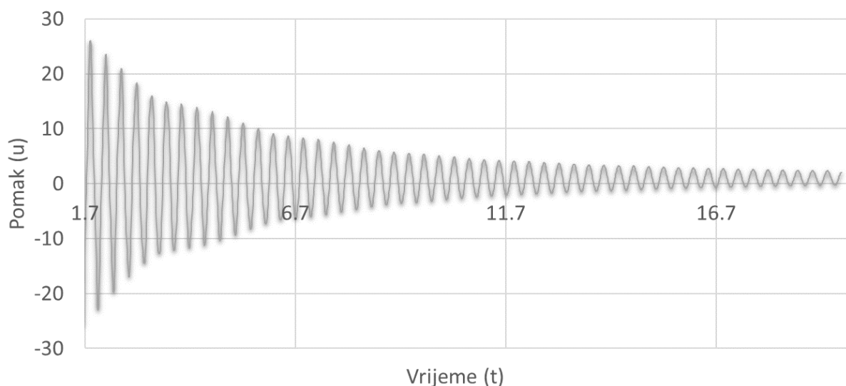
Slika 29. Slobodne prigušene oscilacije 1.ton pomak 1.etaže
