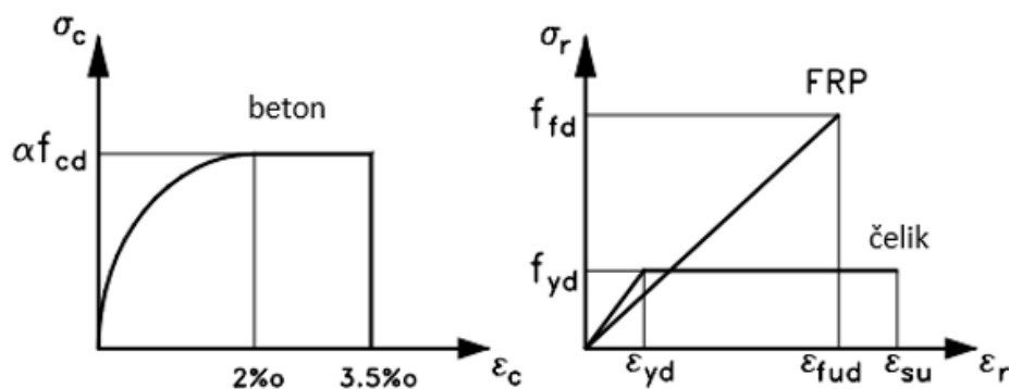
Slika 6: Idealizirane krivulje naprezanje-deformacija konstitutivnih materijala na GSN [1]
