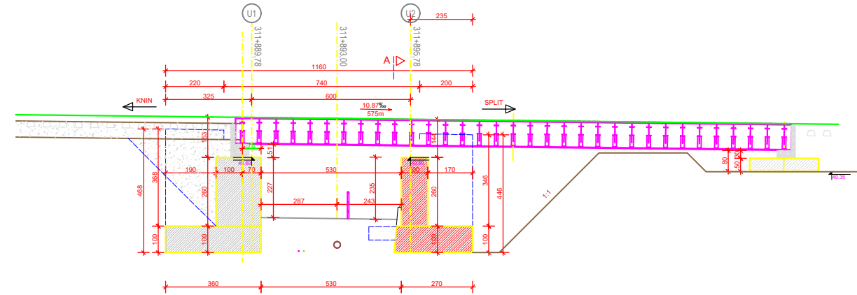
FAZA 1 - provizorij 21 m - pozicija 1 Uzdužni presjek
