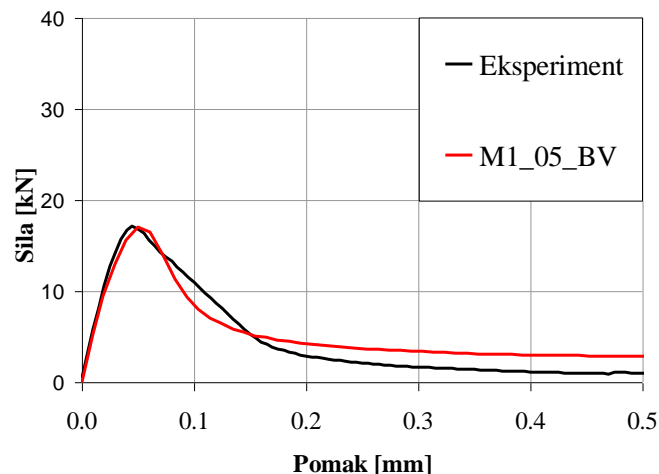
Slika 5.27 Usporedba eksperimentalno dobivenog dijagrama sila-pomak i dijagrama sila-pomak dobivenog numeričkim proračunom za model M1_05_BV
