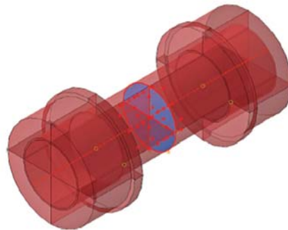
Slika 3.18 Prednapinjanje vijka „bolt load“ tehnikom
