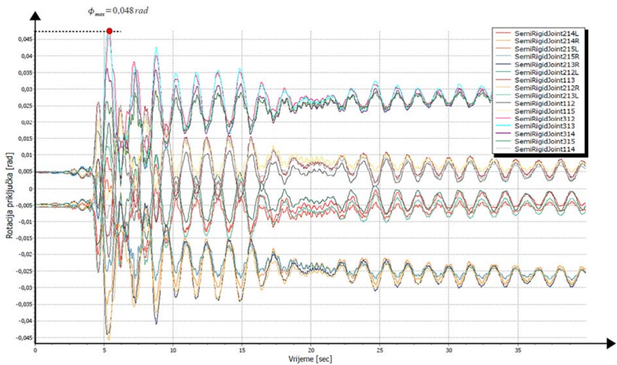
Slika 4.12 Rotacije priključaka u vremenu za okvir s priključcima EP1_3_Richard_Abbott i Loma Prieta potres za vršno ubrzanje od 0,3 g
