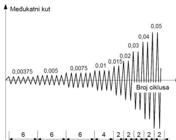
Slika 2.7 Protokol opterećenja (deformiranja) za simulaciju cikličkog djelovanja prema SAC 2000 protokolu [28]
