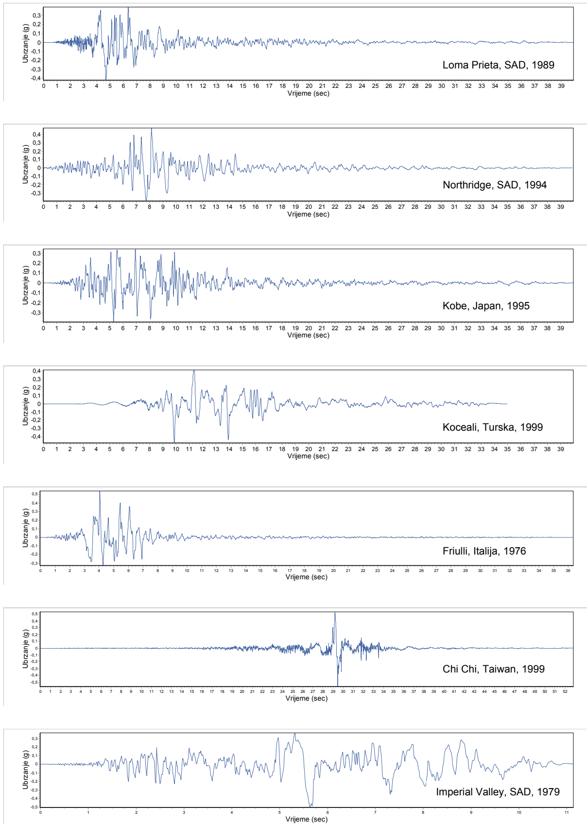
Slika 4.10 Realni zapisi ubrzanja potresa u vremenu podešeni za elastični spektralni ubrzanja za a_g = 0,3g
