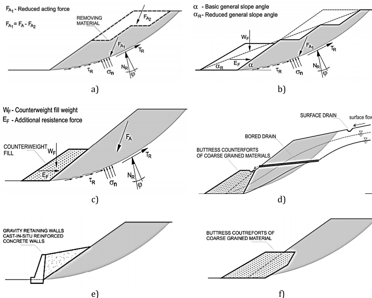
Slika 4: Sanacija klizišta a) uklanjanjem materijala sa gornjeg dijela kosine, b) smanjenjem nagiba kosine, c) dodavanjem protuutega u obliku nasipa, d) kombiniranim dreniranjem, e) izgradnjom armiranobetonskih ili gabionskih potpornih zidova, f) izgradnjom podupirećeg nasipa ili konstrukcijama od armiranog tla [5]
