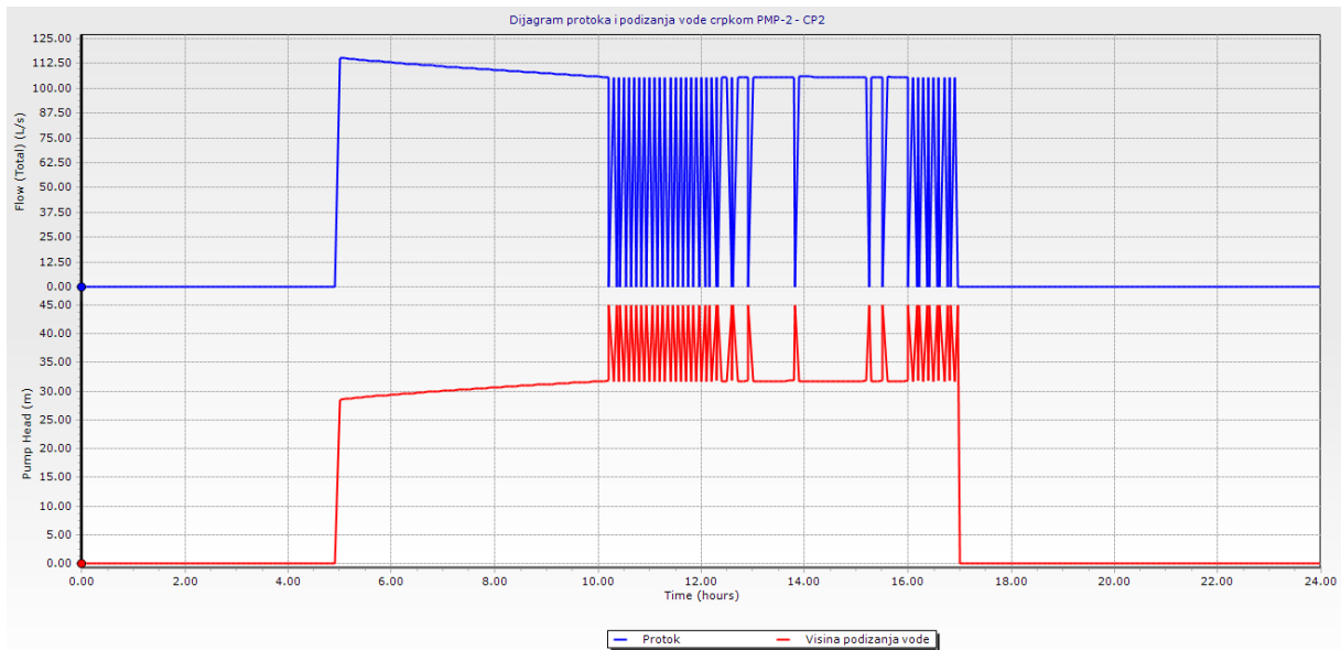
Slika 88. Dijagram protoka i visine podizanja razine vode crpkom PMP-1 – Varijanta 2
