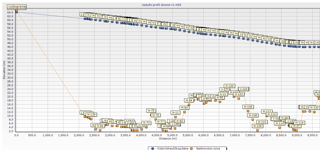
Slika 61. Uzdužni profil dionice vodosprema V1-hotel H29
