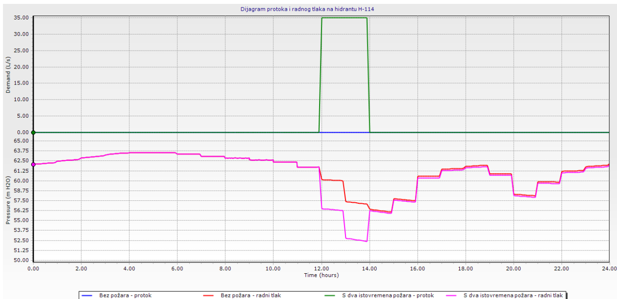
Slika 75. Dijagram radnog tlaka i protoka na hidrantu H-114
