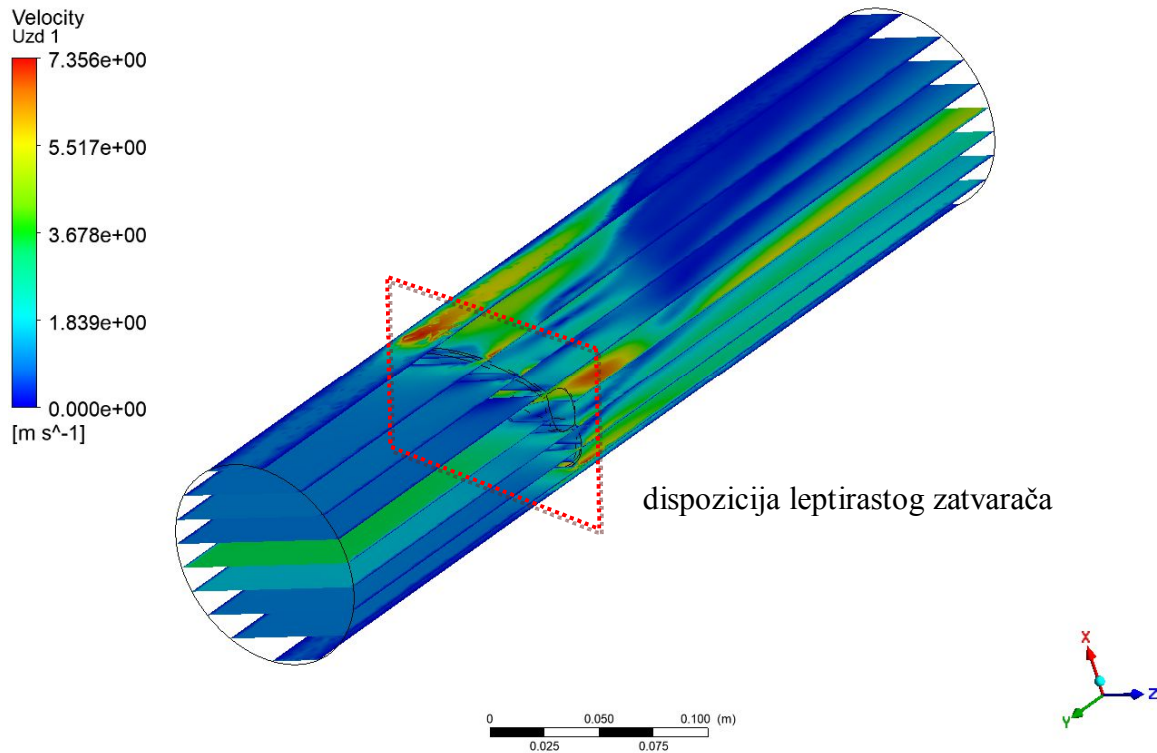
Slika 84. Prikaz položaja uzdužnih profila kod modela leptirastog zatvarača
