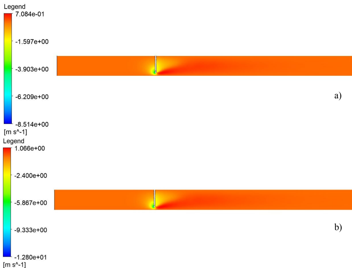
Slika 79. Raspodjela brzina toka u smjeru osi y (brzina v ) na središnjim uzdužnim profilima za podmodel pločastog zatvarača s 80 % zatvorenosti: a) model s ulaznom brzinom toka od 1 m/s, b) model s ulaznom brzinom toka od 1,5 m/s
