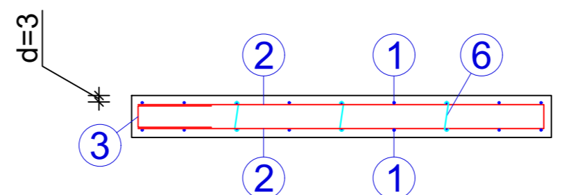
PRESJEK A-A
