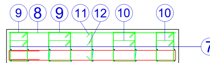
PRESJEK B-B
