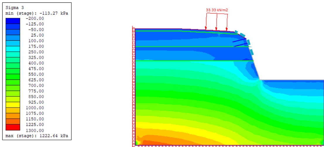
Slika 42 Horizontalna naprezanja za završnu fazu (Opservacijska metoda)
