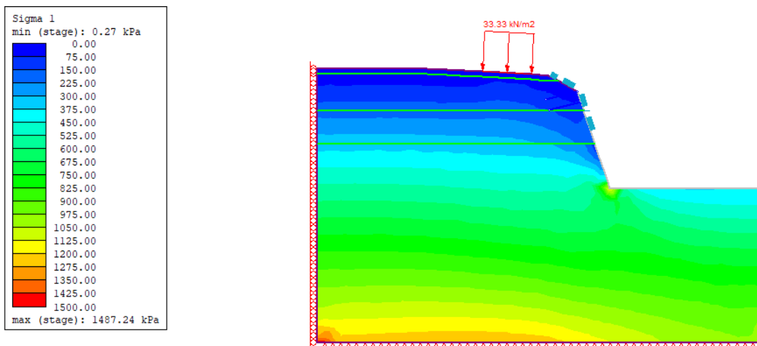
Slika 41 Vertikalna naprezanja za završnu fazu (Opservacijska metoda)
