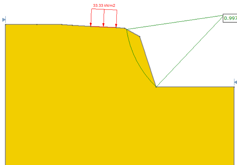
Slika 31 Faktor sigurnosti iskopa (Klasični pristup)
