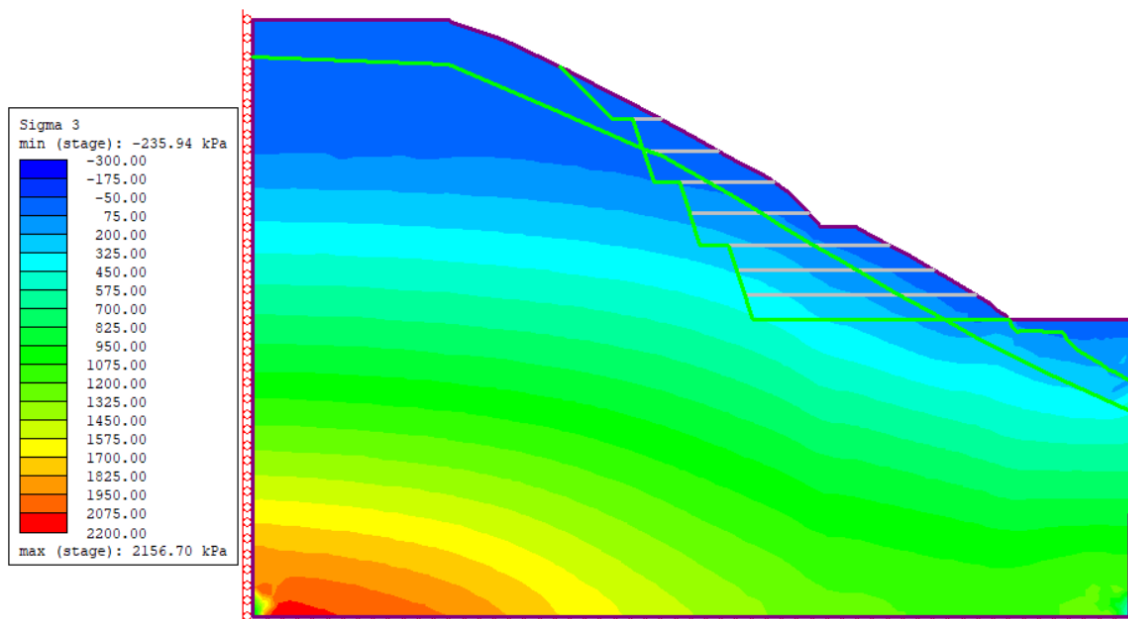
Slika 39 In situ horizontalno naprežanje
